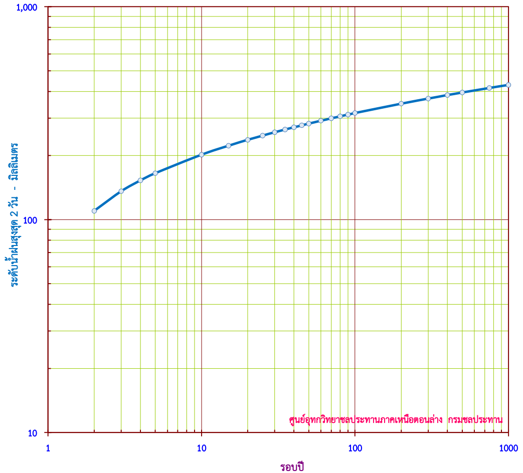
กราฟแสดง ปริมาณน้ำฝนสูงสุด 2 วัน ขนาดรอบปีต่างๆ สถานี 120161 อ.เมือง จ.กำแพงเพชร
